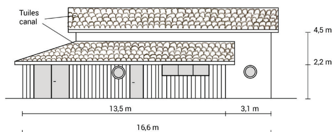
FAÇADE NORD
